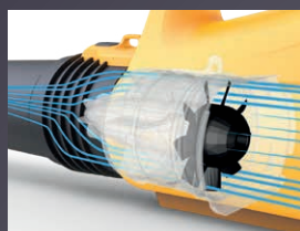
VENTILATEUR AXIAL
